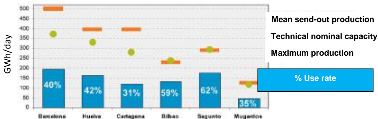
Figure 17. Use rate of LNG terminals in 2009. Source: Enagas
